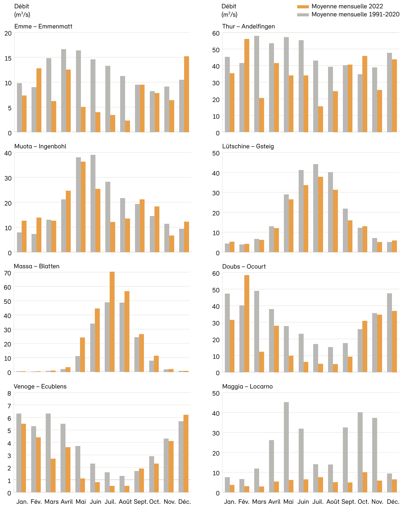
Fig. 4.4 : Moyennes mensuelles 2022 des débits (orange) par rapport à celles de la norme 1991-2020 (gris)
